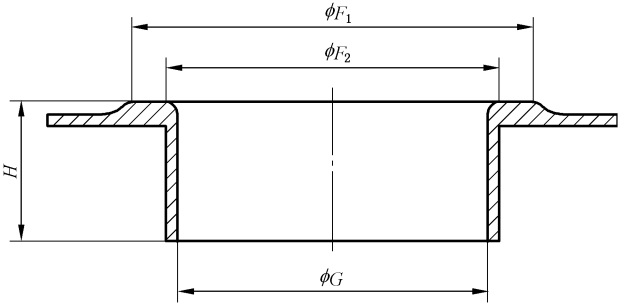
图 L.2 加注孔颈
