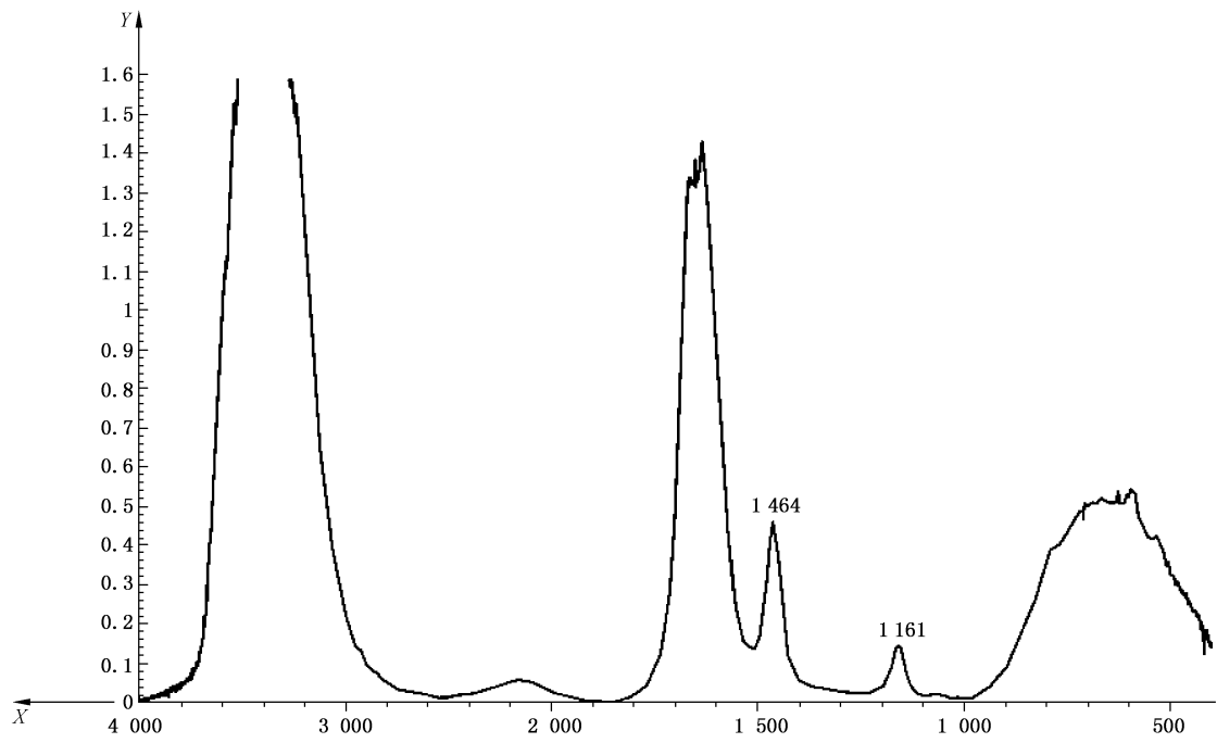
图 H.1 透射法参考谱图
