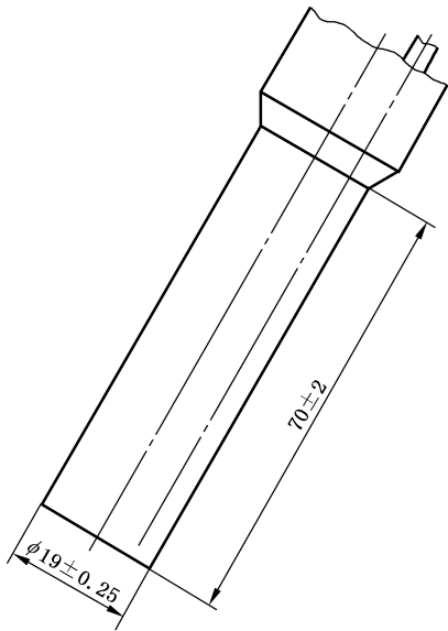
图 K.3 加注嘴
