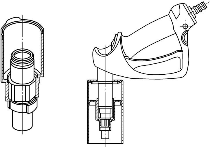
图 L.1 密闭式加注系统实例
