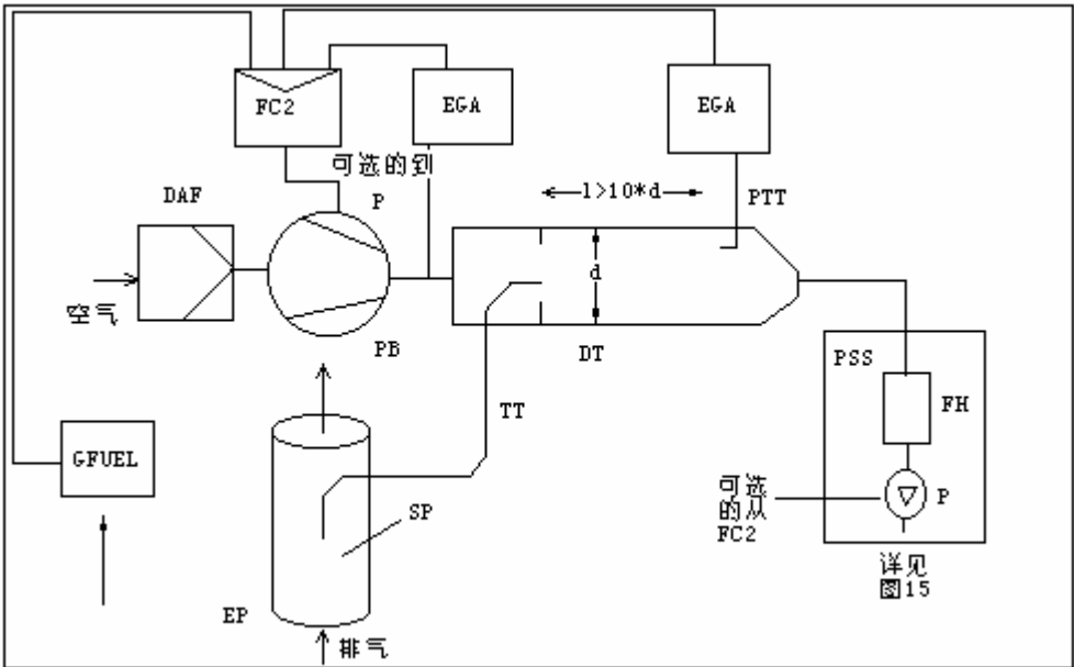
图 7 带 CO 2 浓度测量，碳平衡和全部取样的部分流稀释系统
